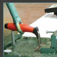
Test de flexion axiale du manche
